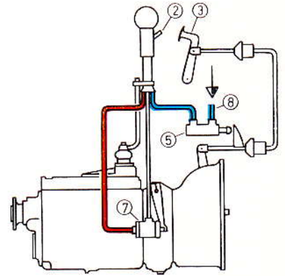
Druckluftschaltung ohne Elektrik Beispiel: Vorschaltgruppengetriebe
