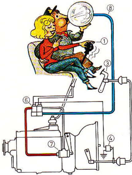
Druckluftschaltung mit Elektrik Beispiel: Vorschaltgruppengetriebe
