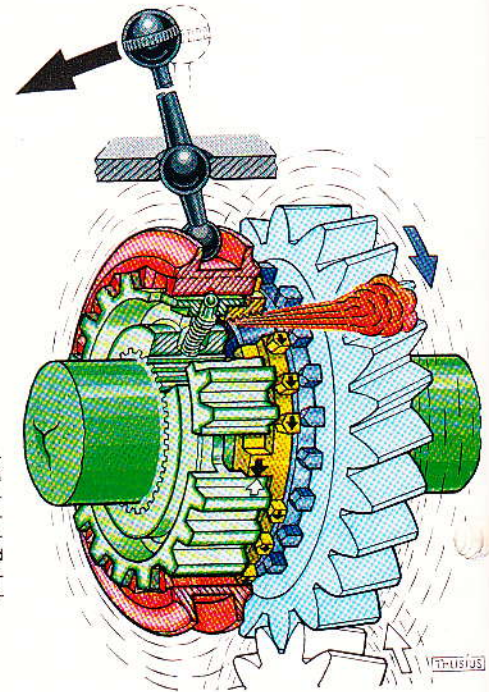
Bild 2 Durch Verschieben der Schaltmuffe wird Synchronring gegen Reibkegel des Zahnades gedrückt. Durch Drehzahlunterschied verdreht sich Synchronring bis festen Anschlag und sperrt Schaltmuffe. Durch ständigen Druck am Schalthebel beginnt Reibarbeit an Kegeln. Braune Rauchfahne!
